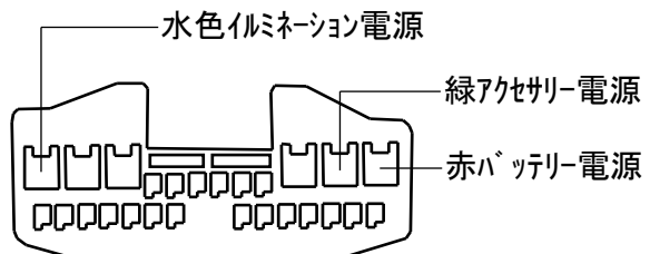
純正オーディオ本体の26Pコネクタを配線側から見た状態
