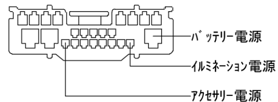
配線側から見た状態
