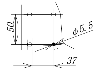
図-1 純正ブラケット右側
